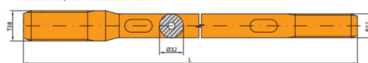
Drifter rod, T38 - Round 32 - R32
