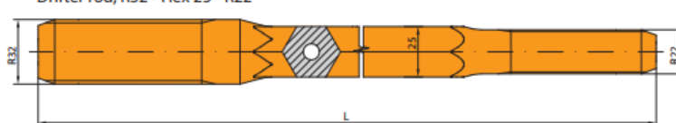
Drifter rod, R32 - Hex 25 - R22
