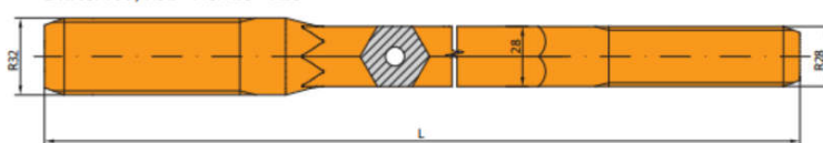
Drifter rod, R32 - Hex 28 - R28
